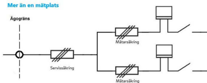
Bild 2. Skiss på anläggning med flera mätarplatser (ex. serviscentral, mätarskåp med flera mätplatser etc.)
