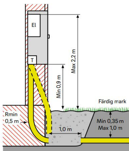
Bild 4. Anslutning av rör mot fasad
