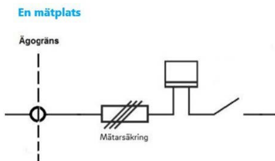
Bild 3. Skiss på anläggning med en mätarplats.
