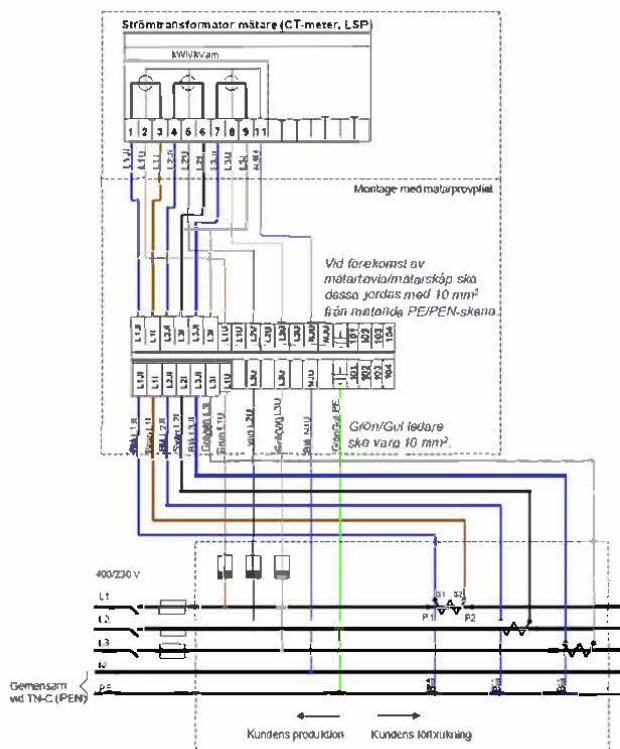
Bild 15. Inkoppling av strömtransformatorer
